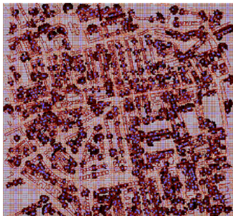
Figuur 3: WiFi-dekking (simulaties) in Notting Hill, Londen op 5GHz, 2.4GHz en in de TV-band. Bron: British Telecom
