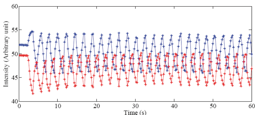
Figuur 8 Gemeten verandering van de fluorescentie-intensiteit onder de elektrodes toen er een blokspanning met een amplitude van 20 Volt tussen de elektrodes werd gezet. De fluorescentie-intensiteit is een maat voor de pH (zuurgraad) van de oplossing.
